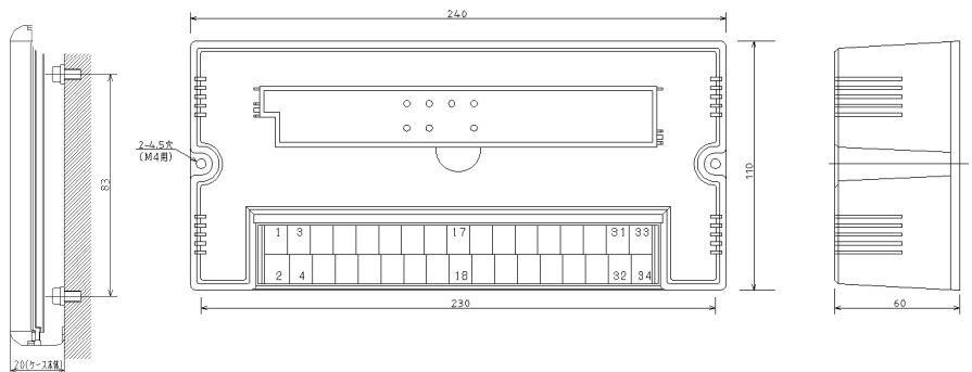
型WK42-RX コントローラ
